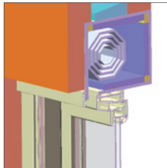
Doorsnede van een in de muur weggewerkte rolluikkast
