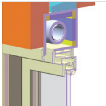
Doorsnede van een in de muur weggewerkte screenkast
