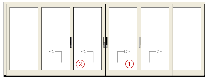
HSP-6L ⑤⑥⑦ ■ hefschuifpui 6 delig
