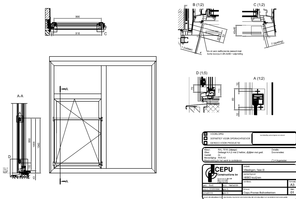
Figuur B4.2 Frans balkon kunststof kozijnen
