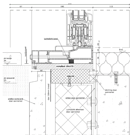
Figuur 5.5 Onderdorpel kunststof hefschuifpui
