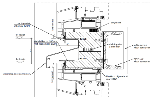
Figuur 9.10 Kunststof horizontale koppeling stalen kolom
