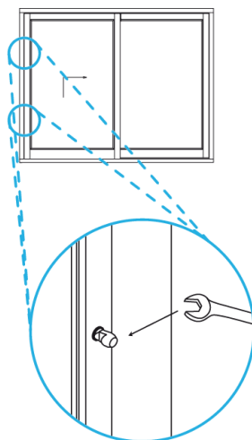
Figuur B2.1 Afstellen hefschuifpui
