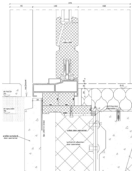
Figuur 5.4 Onderdorpel houten hefschuifpui
