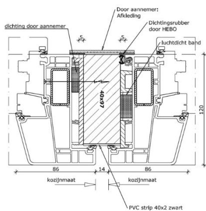
Figuur 9.6 Horizontale koppeling kunststof
