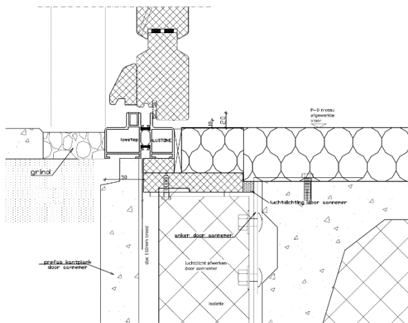
Figuur 7.7 Grind tegen onderdorpel houten kozijn
