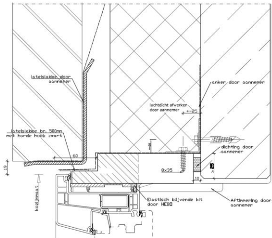
Figuur 7.2 Bovenaansluiting kunststof kozijn
