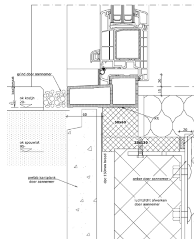
Figuur 7.8 Grind tegen onderdorpel kunststof kozijn
