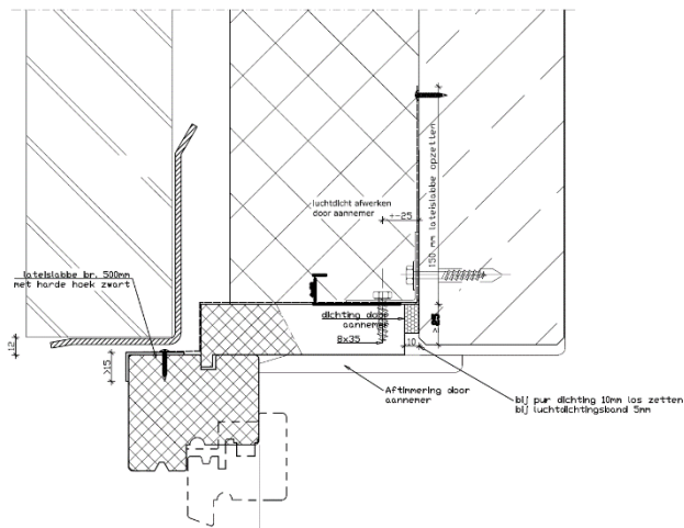
Figuur 7.1 Bovenaansluiting houten kozijn
