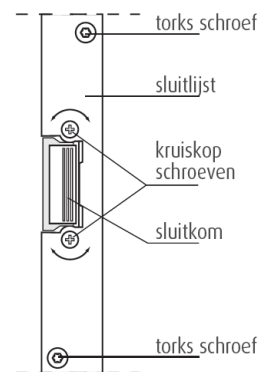
Figuur B1.3 Sluitnokken verstellen
